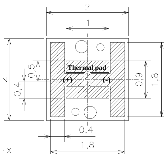
Cu pattern
